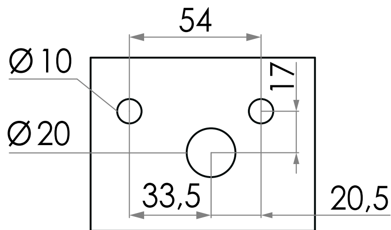
FORATURA COPERCHIO
