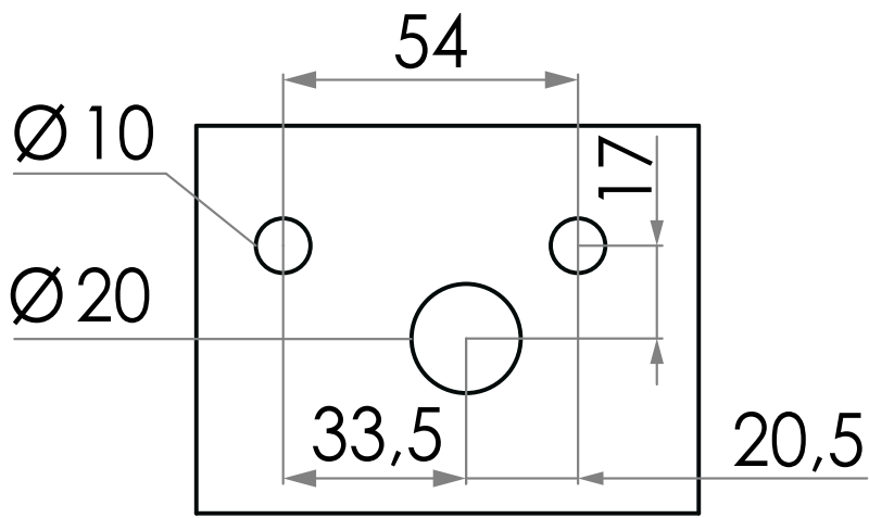
FORATURA COPERCHIO
